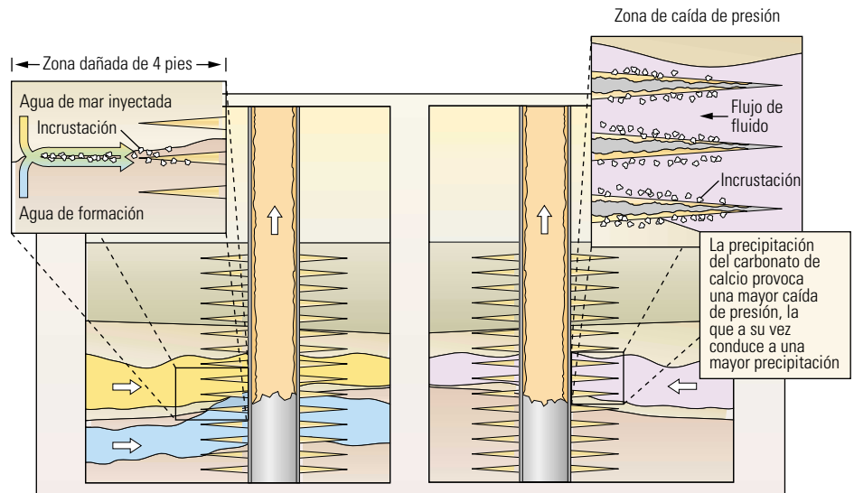
▲ Daños en un pozo en producción. La autosedimentación puede ser causa de problemas en los pozos productivos (derecha), en los que se forman incrustaciones cerca de la garganta de los cañoneos (cuadro derecho). La caída de presión sobre la matriz cercana al pozo puede provocar una precipitación incontrolable de \text{CaCO}_3 . La mezcla de aguas incompatibles (agua de inyección y agua de formación) puede provocar la precipitación de sedimentos minerales en la matriz de la formación (izquierda).
