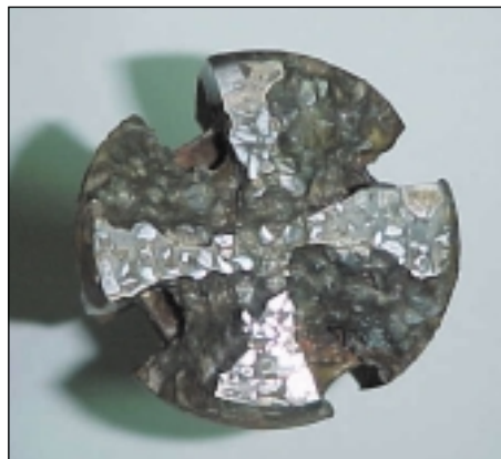
▲ Cabeza pulidora gastada por el polvo de sílice.
