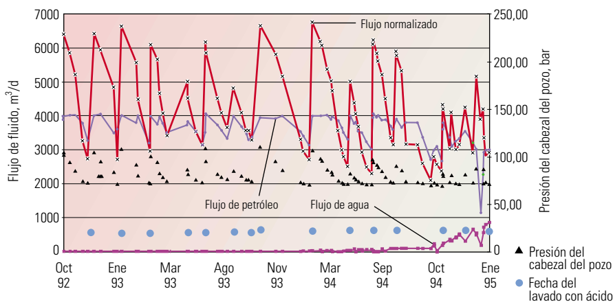
▲ Perfiles de producción serrados. Esta porción de la historia de la producción correspondiente a uno de los pozos prolíficos del campo Gullfaks muestra un deterioro cíclico de la producción. El flujo normalizado (curva roja) es un buen indicador de los cambios de productividad debidos a los esfuerzos de intervención, ya que elimina los efectos de estrangulación de la producción provocada por las limitaciones del equipo de superficie. La curva normalizada muestra el gran impacto ocurrido en forma inmediata como consecuencia de los distintos tratamientos ácidos (indicados por los círculos azules) y la consiguiente pérdida en la productividad del pozo, que se produce de uno a tres meses más tarde, lo cual indica la presencia recurrente de precipitaciones minerales.
