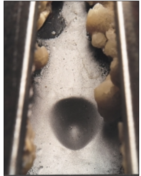
▲ Eliminación de incrustaciones de carbonato de calcio con chorro de agua abrasivo. La tubería recibió un solo chorro de agua con arena abrasiva a razón de 2,4 pulg./min [1 mm/seg]. Durante el ensayo se mantuvo el chorro en la misma posición durante 3 minutos, y el chorro de arena penetró casi el 80% de la pared del tubo (nivel de daño inaceptable).
