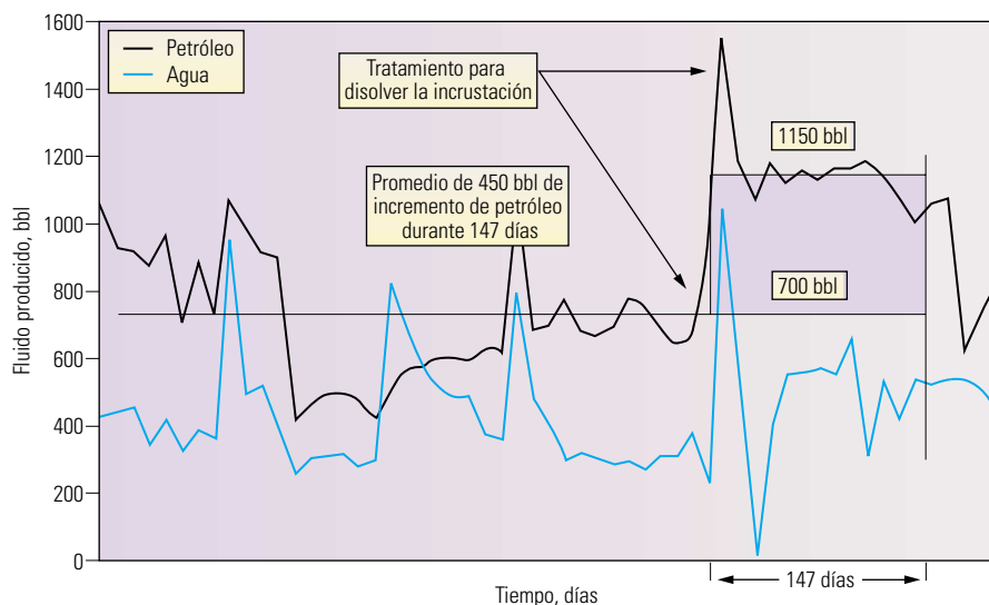
▲ Historia de producción de un pozo en el Mar del Norte. Se observa un elevado nivel de daño debido a incrustaciones de \text{BaSO}_4 y \text{CaCO}_3 en los cañoneos y en la matriz cercana al pozo, que fue tratado con éxito, como resultado de lo cual se obtuvo un incremento del 64% en la producción de petróleo durante más de 147 días.
